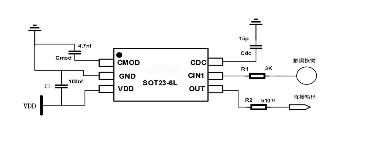
图 3-1 ： 应用电路
