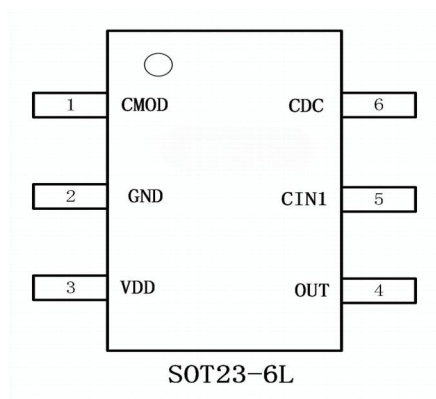
图1-1: 封装简图
