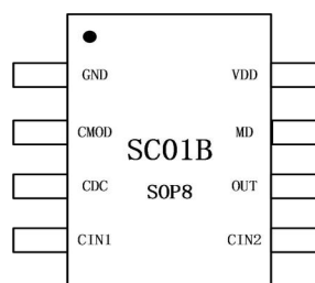
图1-1： 封装简图
