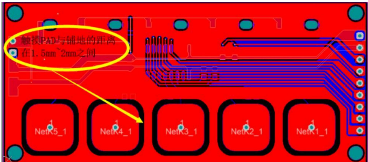
图 7-1：触摸 PAD 离铺地 1.5MM 以上
