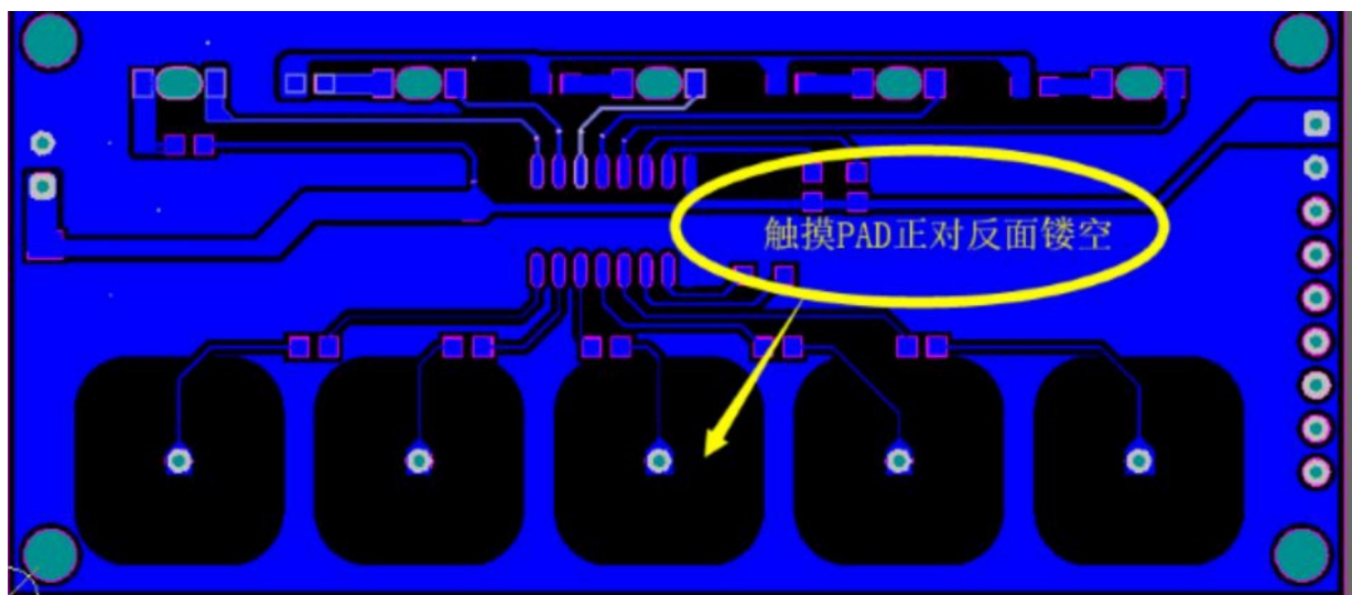
图 7-2：触摸 PAD 正背面镂空
