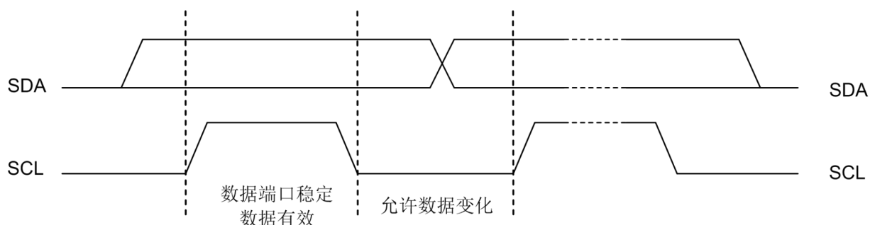
图 3-7 : 数据有效
