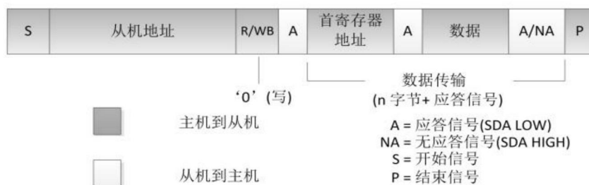
图 3-8 : 写操作
