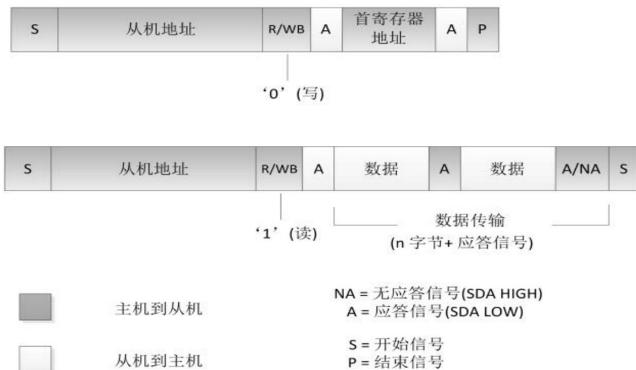
图 3-9 : 读操作
