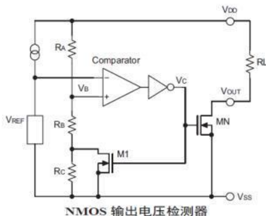
NMOS 输出电压检测器
