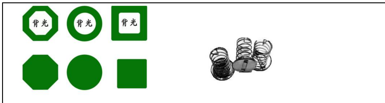
按键感应盘可以是实心或中空矩形、圆形，多边形
