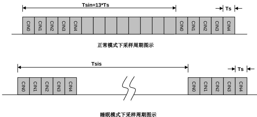
图 2-1：正常和睡眠模式下采样周期图示
