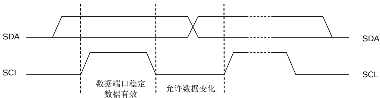
图 3-7 : 数据有效
