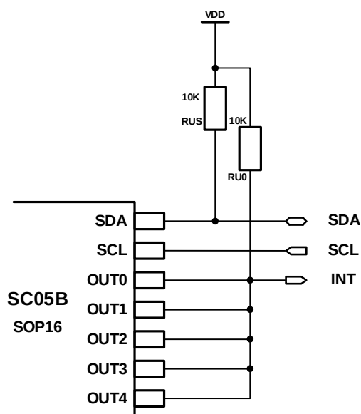
图 3-4: I 2 C 中断方式
