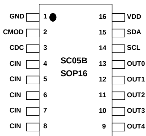
图 1-1: 封装简图
