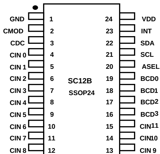
图1-1: 封装简图
