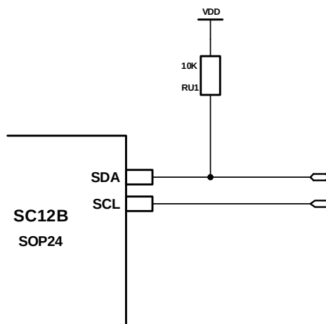
图 3-4 : I2C接口
