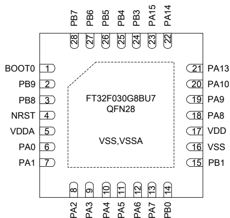
图 4-10 QFN28(B)引脚分配
