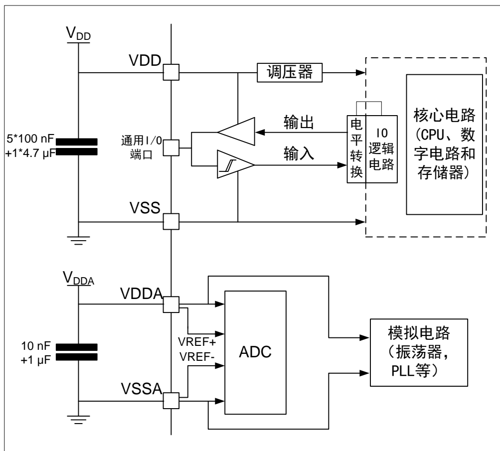
图 6-3 供电方案图
