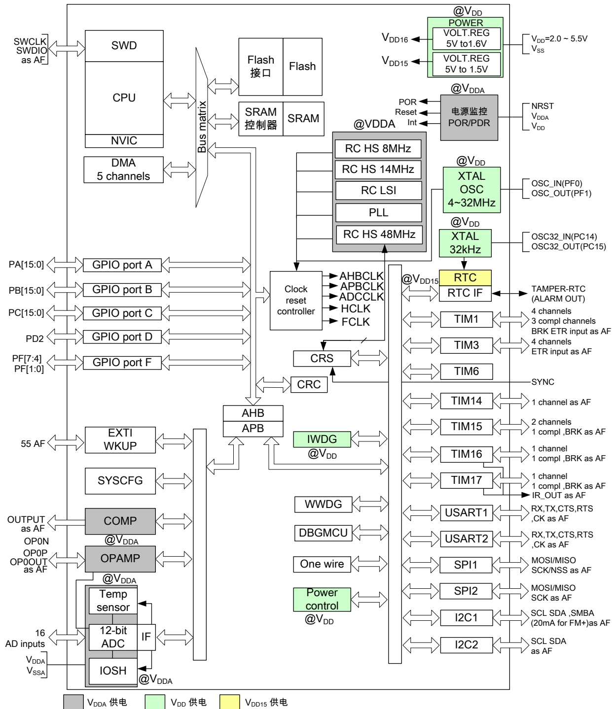
图 2-2 系统框图
