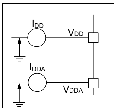
图 6-4 电流消耗测量方案
