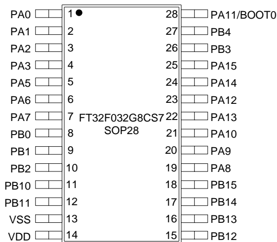
图 4-6 SOP28(C)引脚分配
