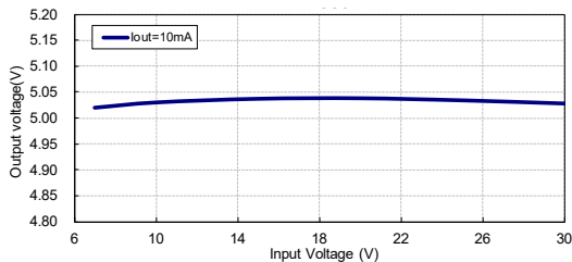
输出电压与输入电压: HT7550-1
