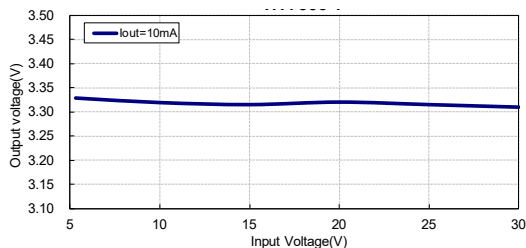
输出电压与输入电压: HT7533-1
