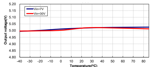
输出电压与温度: HT7550-1
